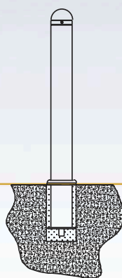
Montaż do podłoża przez zabetonowanie futerału
