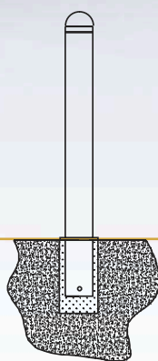
Montaż do podłoża przez zabetonowanie rury kotwiącej
